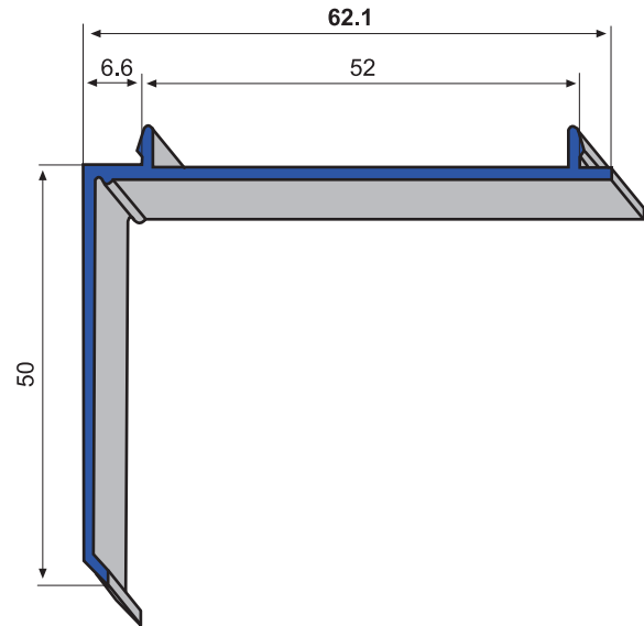
C/ 221 Tapajuntas forro - 50
