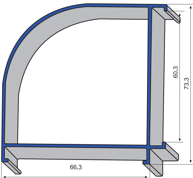
C/ 314 Esquinero de 45ª
