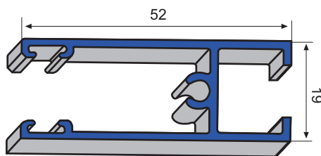
C/ 110 Hoja de rueda cristal -10
